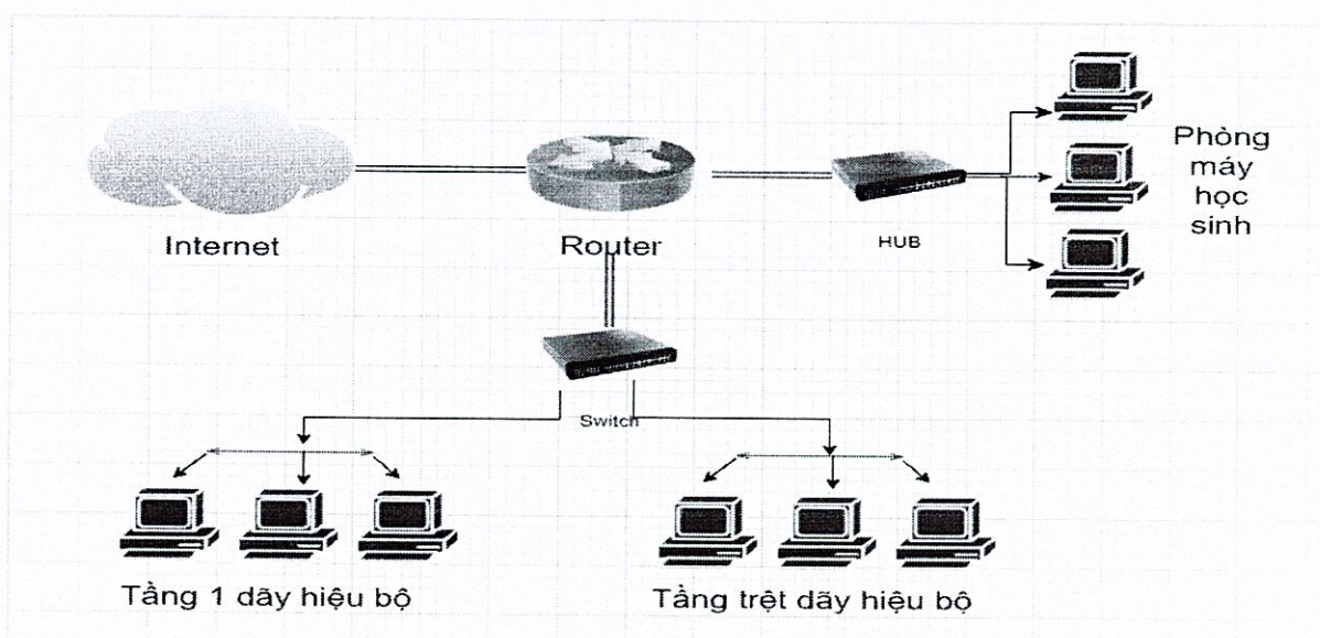
Hình 2: Sơ đồ kết nối vật lý tổng thể hệ thống mạng trường THPT Minh Long
